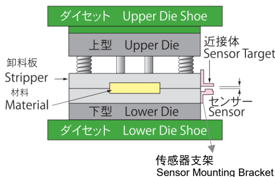
安装于模具的示意图 Installation drawing
