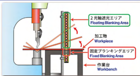
フィックス+フローティング・ブランキング機能 Fixed + Floating Blanking
