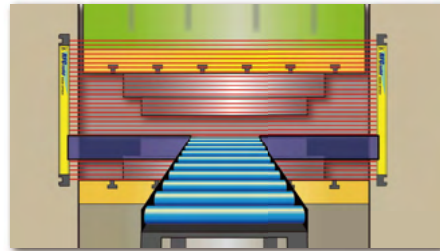
フィックス・ブランキング機能 Fixed Blanking
