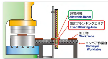
許容光軸付きフィックス・ブランキング機能 Fixed Blanking Function with Allowable Beam
