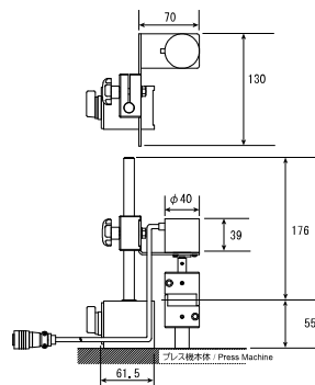
直結タイプ / Direct-coupled type encoder (Model: SDM3-C)
