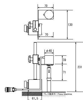
押し付けタイプ / Pressing type encoder (Model: SDM3-O)
