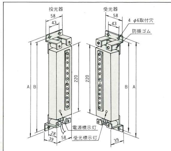
フロント型(Fタイプ) Sタイプも同寸法
