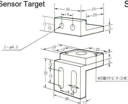
型式 Model JMKS-1
